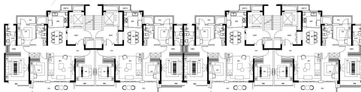
小高层7/8#平层图
