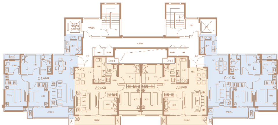
1#平层图
