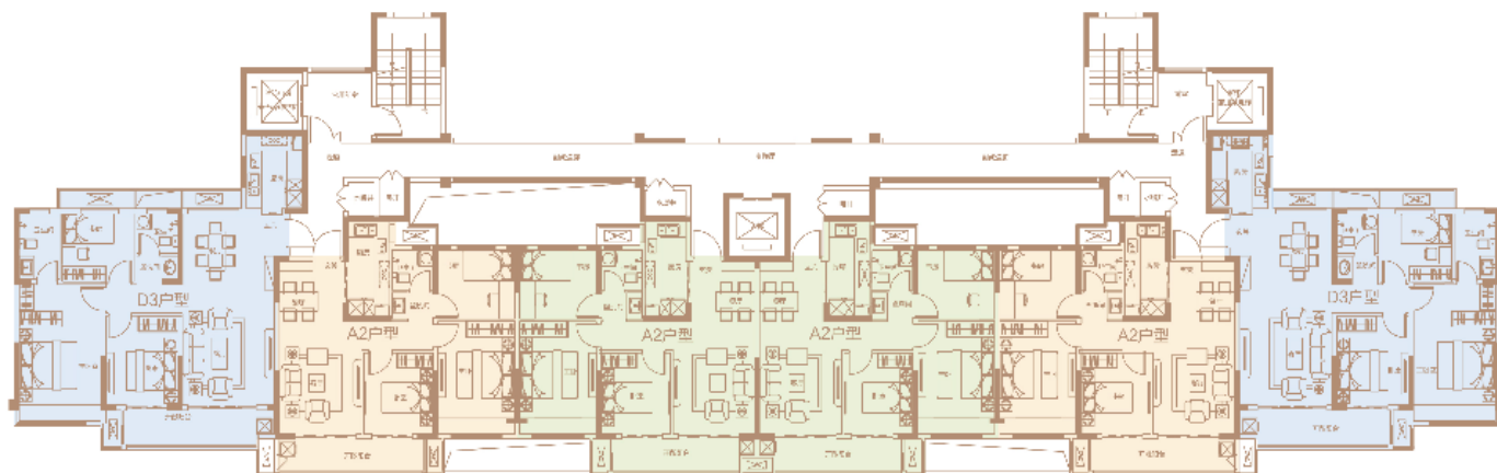
6#平层图
