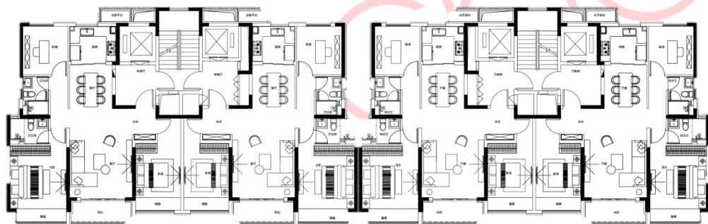
小高层2#平层图
