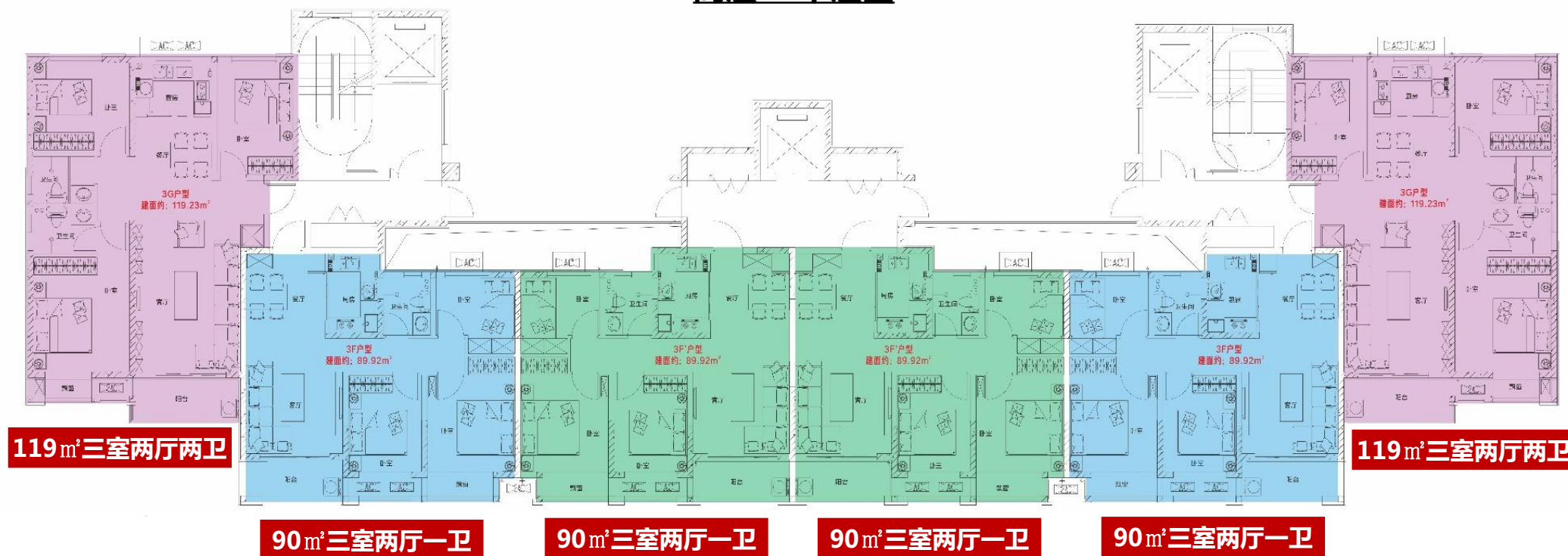
高层5#平层图
